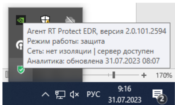
Рисунок 5 – Агент верифицирован
